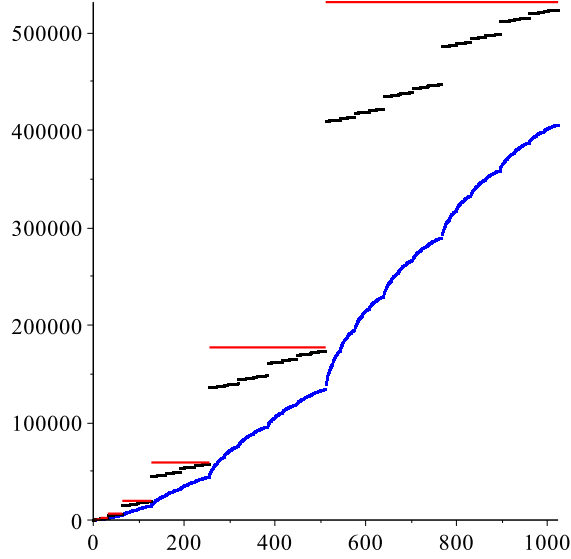
FIGURE 1. Comparaison des graphes de la complexité ( u_n ) dans l'algorithme de Karatsuba (en bleu ), de la suite majorante ( v_n ) (en noir) et la suite super majorante ( w_n ) (en rouge ) (exemple 26).
